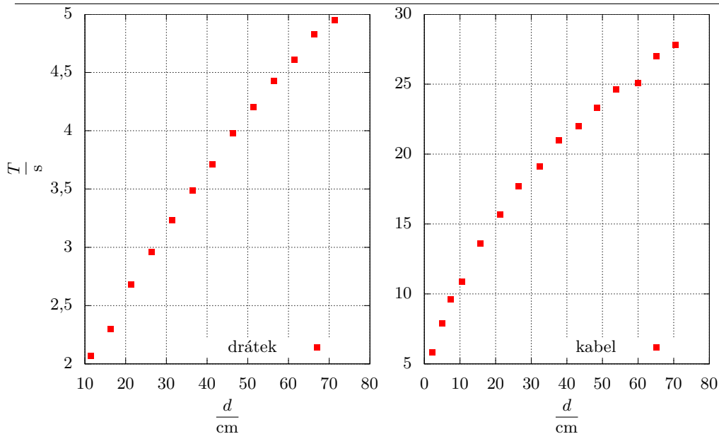
Obr. 1: Závislost periody kmitu tyčky na délce závěsu pro obě lanka. Všimněme si rozdílných rozsahu os.
