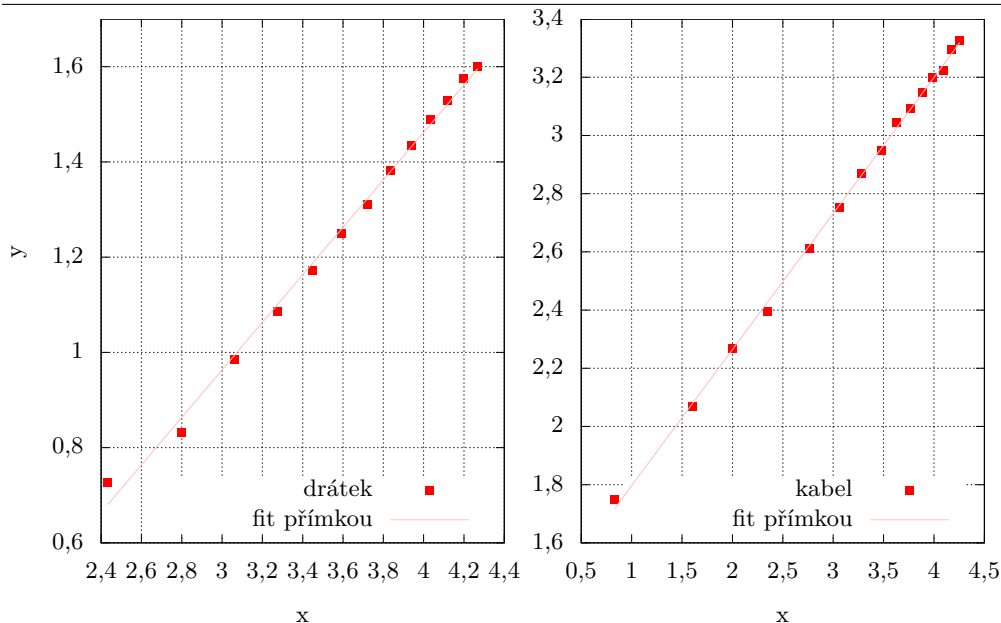
Obr. 2: Závislost logaritmu periody kmitu tyčky na logaritmu délky závěsu pro obě lanka. Všimněme si rozdílných rozsahů os.
